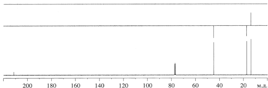
Спектр А
