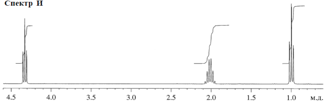
Спектр И
