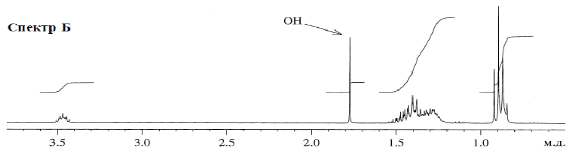
Спектр Б
