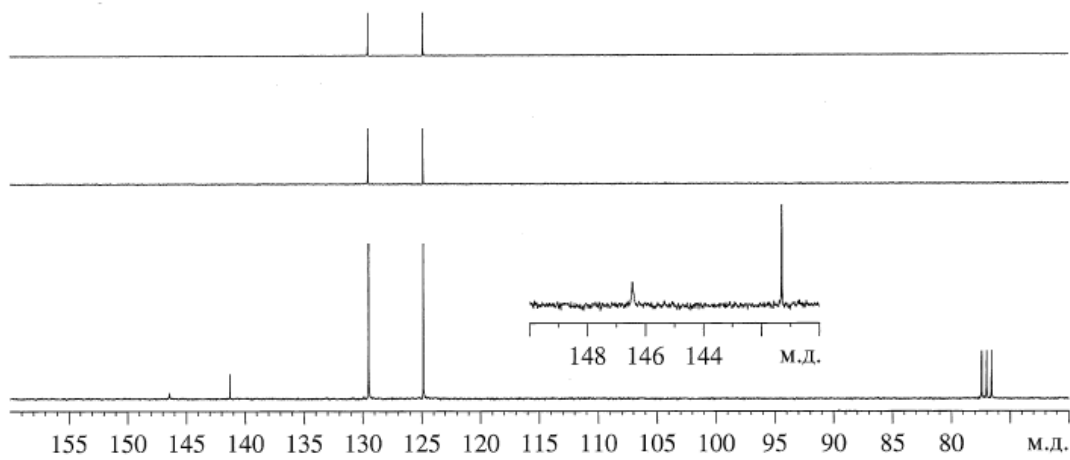
Спектр P
