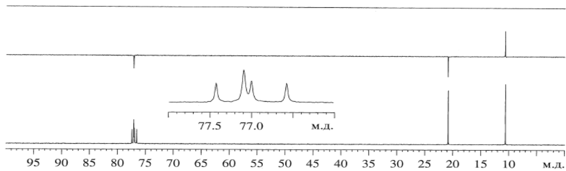
Спектр И
