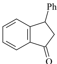
3-фенилиндан-1-он
