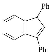
1,3-дифенил-1H-инден
